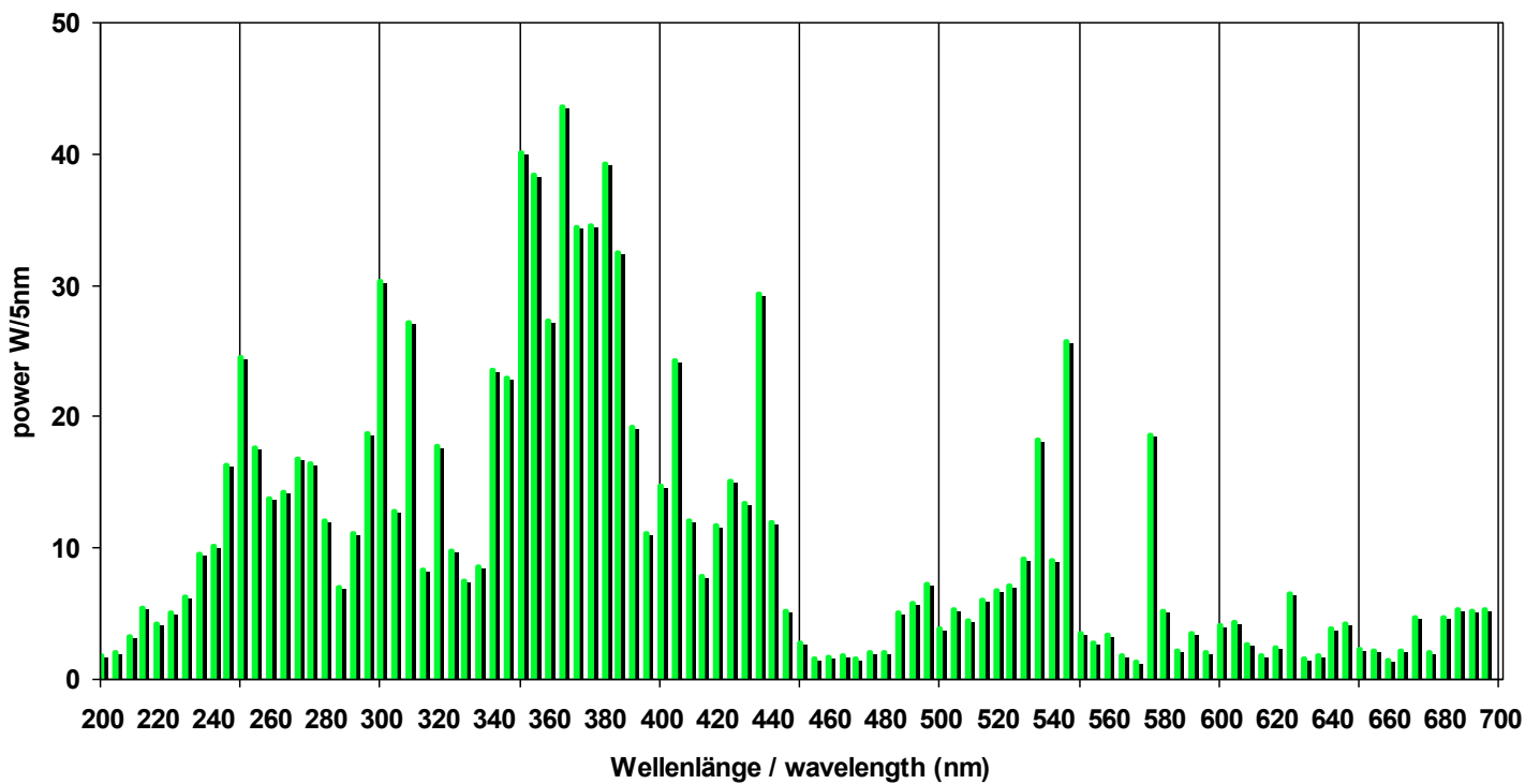
Spektrum Eisen / Iron Fe 100 W/cm
